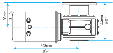
V2/3 Gruppo motore/riduttore (senza sistema FastFit)
