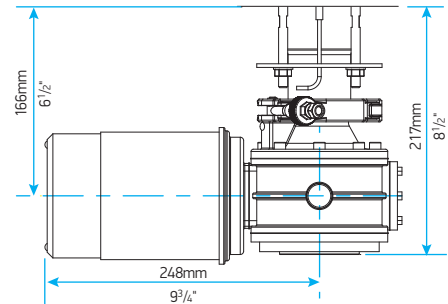
V2/3 Gruppo motore/riduttore (con sistema FastFit)
